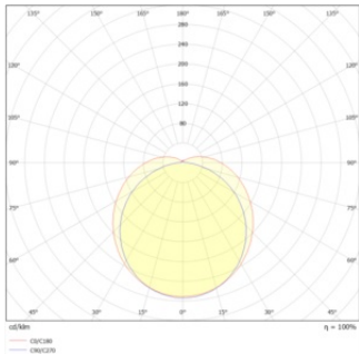
DP 3TH 600 E 17W 857 IP65 GY
